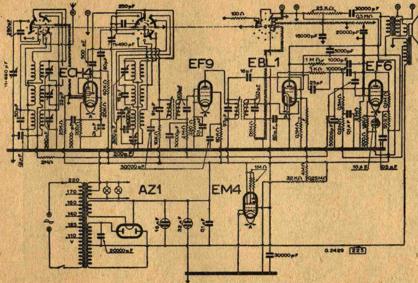
Lo schema elettrico dei ricevitori Philips modd. « 666 » « BI 560/A » « BI 561/A ».
